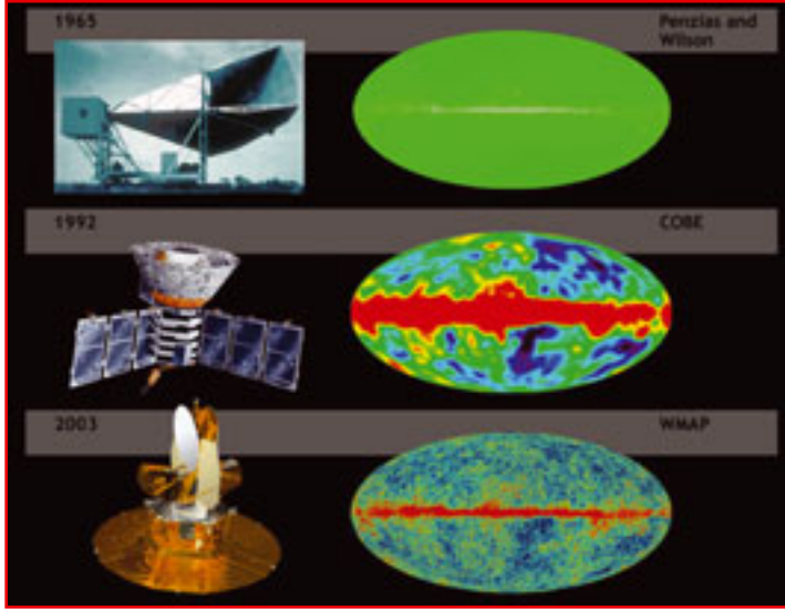
Big Bang'in en büyük kanıtlarından biri olan kozmik arka plan dalgalanmaları 1965 yılında keşfedilmiştir ve ayrıca COBE (1992) ve WMAP (2003) uzay uydularınca incelenmektedir.
