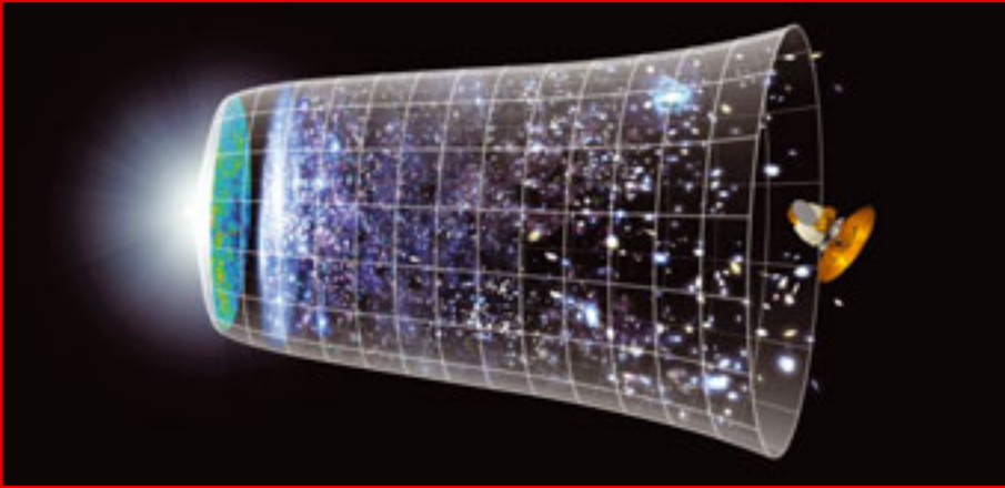
2006 yılında WMAP uydusu verileriyle hazırlanan bu grafik, Big Bang'in ilk döneminden günümüze kadar evrenin genişlemesini temsil ediyor.
